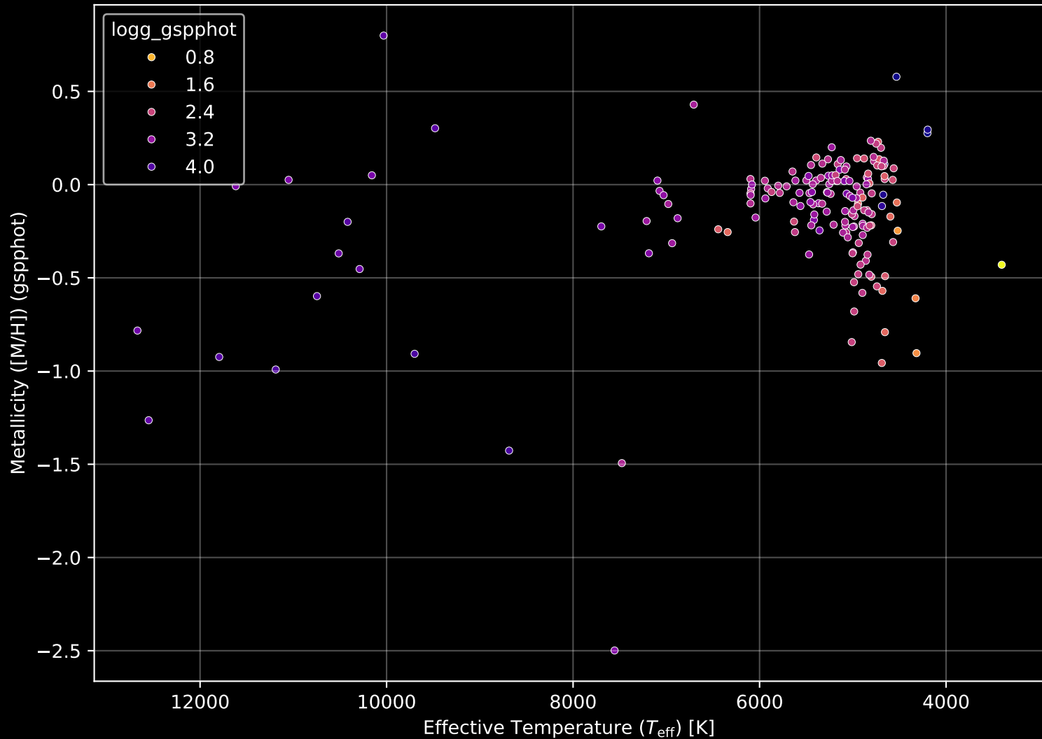
APOGEE DR17 Field: [113-04] Stellar Population Parameters (n= 176)
